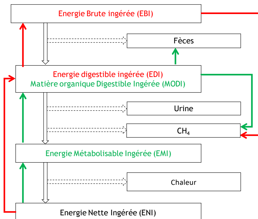
Figure 32 : Schéma comparatif de la méthode de la méthode MONDFERENT I (vert) avec la méthode Giec 2006 (rouge)
